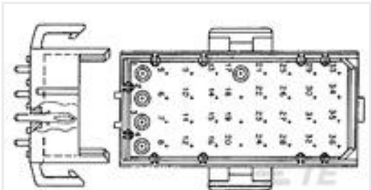
TE 产品编号2-640506-4 36P MR HDR ASSY VO LF
