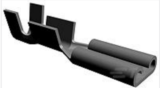
TE 产品编号61454-1 WRAP TYPE TAB RECEPTACLE 24-20 AWG TPBR
