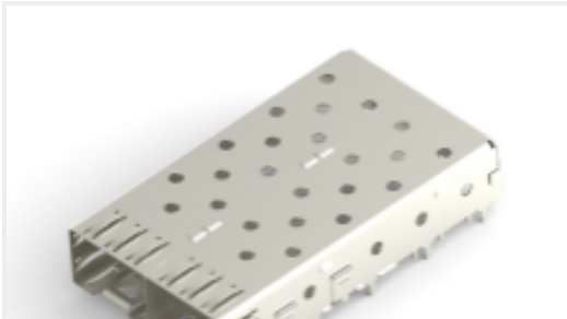
TE 产品编号1761014-3 SFP 1X2 CAGE ASSY, PRESS FIT
