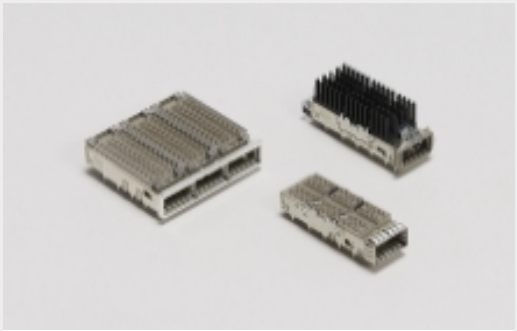
QSFP、QSFP+ 和 zQSFP+(142)
