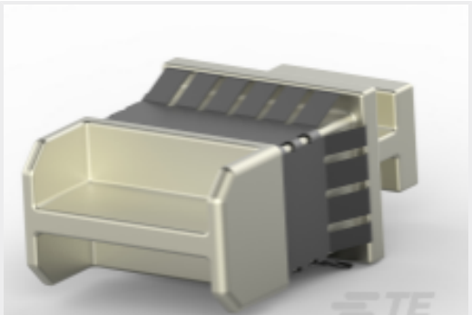
TE 产品编号 1888901-1 SFP+ EMI Plug
