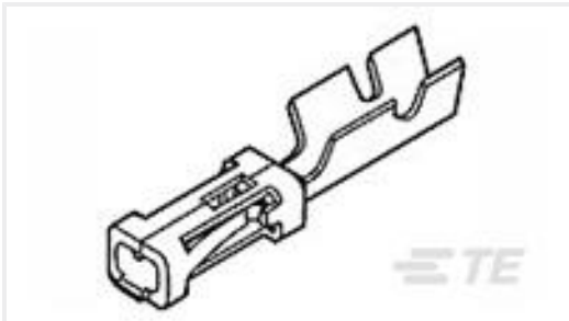
TE 产品编号5-102316-6 MOD IV RECP PLTD 15 DPLX LF
