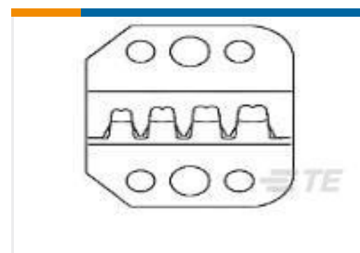
TE 产品编号 58541-2 PRO-CRIMPER HAND TOOL DIE
