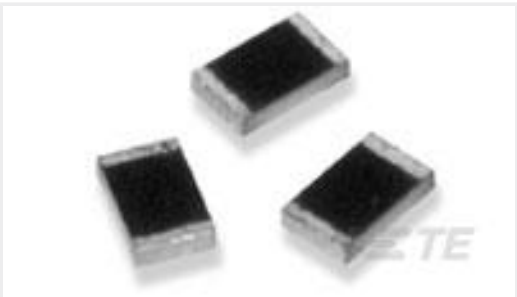
TE 产品编号2-1625868-1 RP 2A 0.25W 2K0 0.1% 25PPM 1K RL
