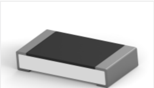
TE 产品编号9-2176388-9 RQ 1206 105R 0.1% 10PPM 5K RL
