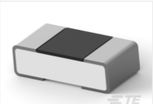
TE 产品编号9-2176363-3 RQ 0402 3K92 0.1% 10PPM 5K RL
