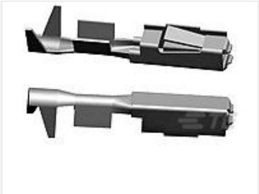
TE 产品编号144969-2 MQS0,63 Au rec LL unseal. 0,2-0,6
