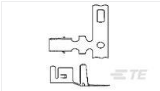
TE 产品编号3-647334-1 MINI AMP-IN 2000,14-18 AWG LF
