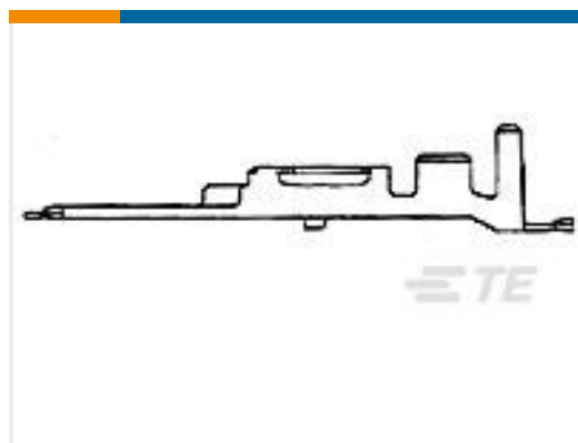
TE 产品编号172778-1 MIC MK-2 TAB LP
