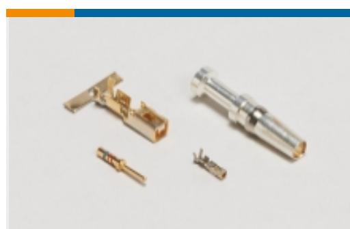
连接器端子(27)
