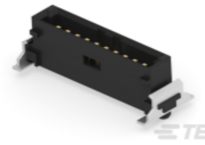
TE 产品编号294919-E SRCP 1,27 10 M 1 SMD 137 E1 094 * GU-H *
