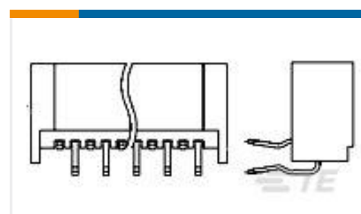
TE 产品编号 2-1734803-8 FPC Non Zif 1.25mm 28P R/A
