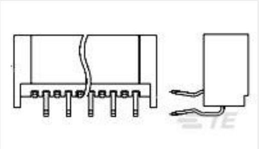
TE 产品编号 2-1734803-0 FPC Non Zif 1.25mm 20P R/A
