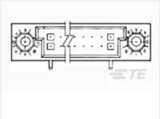
TE 产品编号1-532428-4 HDI RECP ASSY 2 ROW 150 POS
