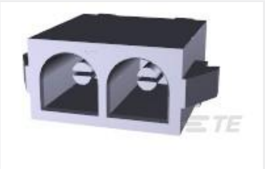
TE 产品编号350582-4 02P UMNL PIN HDR ASSY V2 LF
