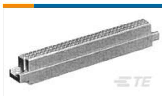
TE 产品编号925486-1 MOD. IV SNAP-IN HSG 96 POS.
