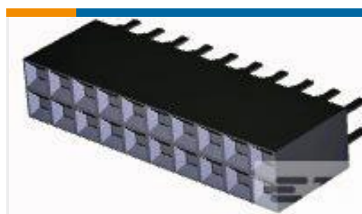
TE 产品编号1-534206-0 20 MODII VRT DR CE 100/115
