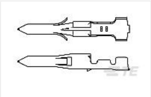
TE 产品编号794018-1 .062 CP&S PIN PTPBR L/P 30-24
