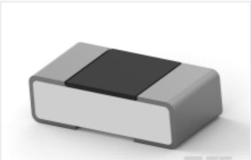
TE 产品编号4-2176360-7 RQ 0402 1K3 0.1% 10PPM 1K RL
