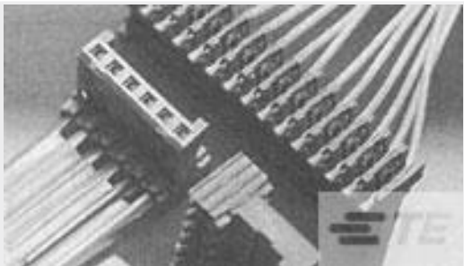
TE 产品编号281709-8 PLUG HE13 IDC 90 8 P AWG 24
