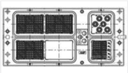
TE 产品编号2101882-2 A600R,Sz2,150/85/150/150/Q6,CHRM,FR.250
