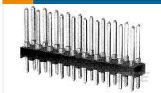
TE 产品编号 1-87227-4 28 MODII HDR DRST UNSHRD .100
