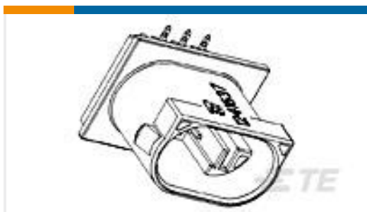
TE 产品编号 1241637-1 6pos MQS .63 header 90deg
