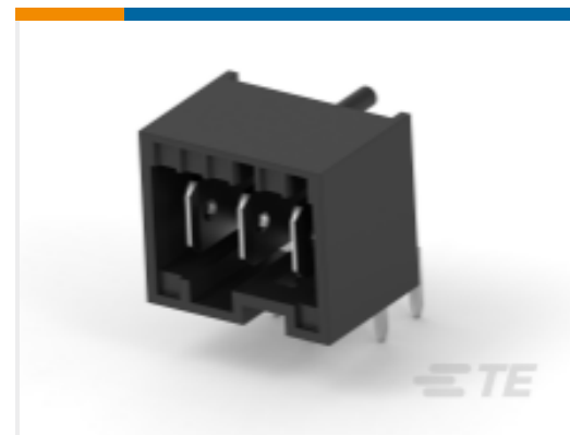
TE 产品编号 1-521384-3 ASSY PL R/A RAST5 HEADER 03-B
