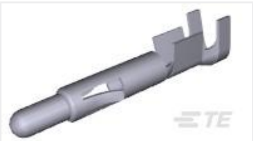
TE 产品编号1903116-2 DYNAMIC D1000 TAB CONT AU 0.38 um M L/P
