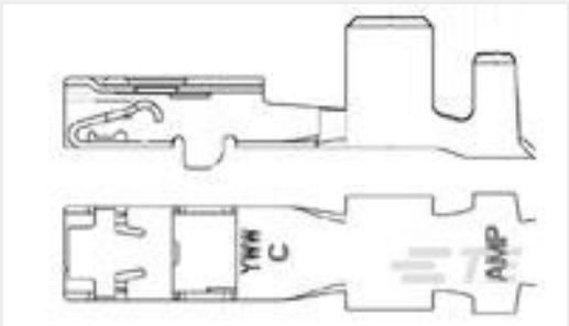
TE 产品编号1326030-4 2.8MM RECP,UNSEAL,10-12AWG
