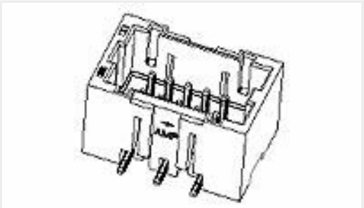
TE 产品编号 9-292229-0 1.5 MINI CT D/R SMT 40P V ONTA
