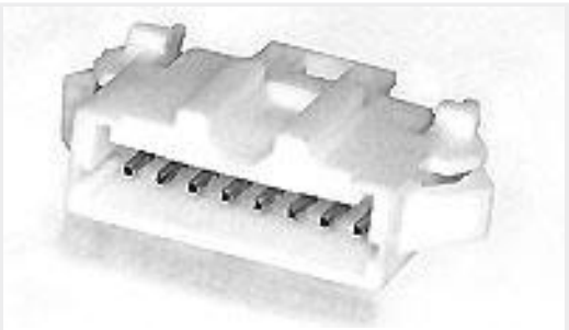
TE 产品编号 7-292215-0 MINI CT SGL RELAY 20P BLUE
