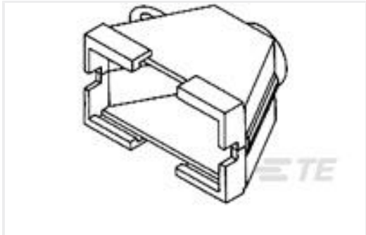
TE 产品编号350374-1 12P STR/REL HSG HNGD V0
