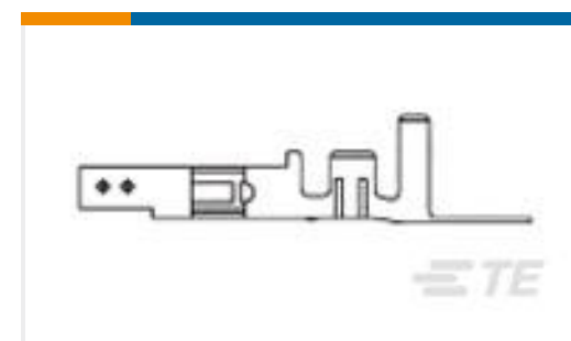
TE 产品编号794956-4 VAL-U-LOK SKT PHBZ AU 22-18AWG
