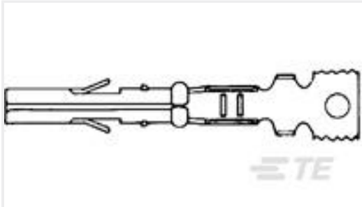
TE 产品编号641294-2 MR RECPT 26-18 AUNI/AUPHBZ
