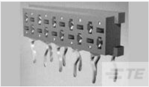
TE 产品编号 9-100400-0 MICRO-MATCH FSID NP
