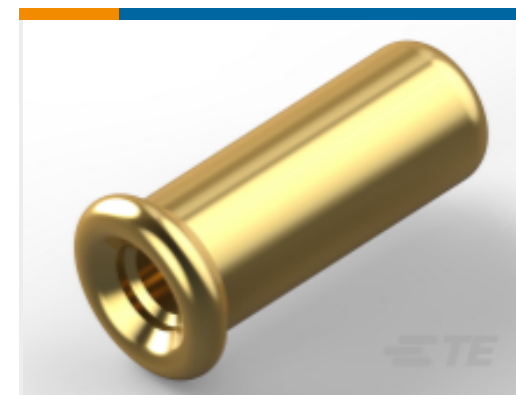
TE 产品编号50863-4 微型弹簧插座：底部闭合，镀铜，4A
