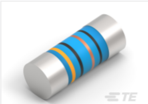
TE 产品编号9-2176316-8 MELF SMA-A 680K 1% 50PPM 0207 1W
