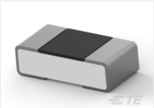
TE 产品编号1-2176364-8 RQ 0402 6K98 0.1% 10PPM 5K RL
