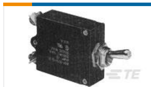
TE 产品编号4-1393247-4 W31-X2M1G-7.50=W23/W31
