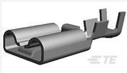
TE 产品编号175022-1 250 PL EX REC. 18-14AWG PTBR
