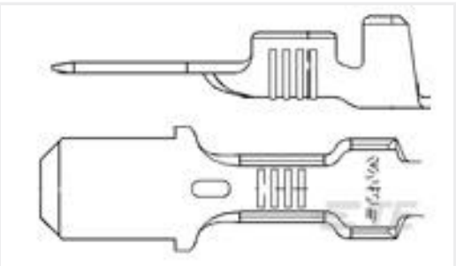
TE 产品编号63857-1 FASTON 187 TAB 22-18 AWG TPBR
