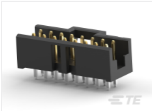
TE 产品编号 2-2823933-6 26P,2MM,PL HDR,DRVT,2.2,0.38AU,TB W/CAP
