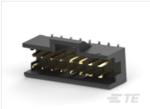
TE 产品编号 2-2823244-0 20P,2MM,PL HDR,DRV,T,SMD,0.76AU, TR W/CAP
