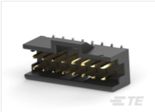
TE 产品编号 2-2823240-0 20P,2MM,PL HDR,DRV,T,SMD,0.38AU, TR W/CAP
