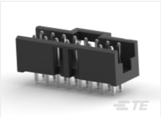
TE 产品编号 2-2823538-0 20P,2MM,PL HDR,DRV,T,2.8,SN,TR W /CAP
