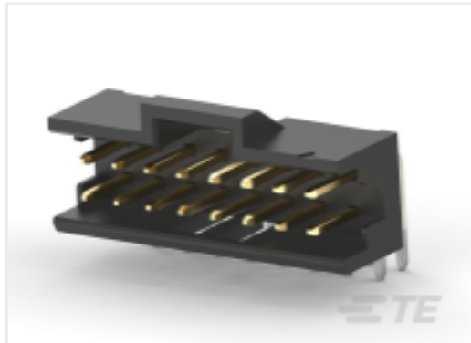
TE 产品编号 2-2823228-0 20P,2MM,PL HDR,DRRT,2.2,0.38AU,TB
