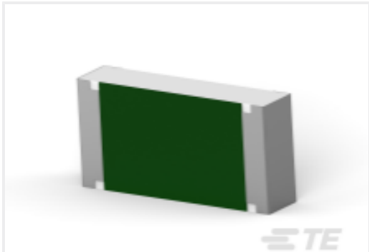
TE 产品编号4-2176397-1 3502 47R 1%
