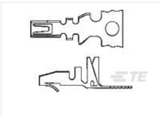
TE 产品编号3-794121-1 TERMINAL, MINI AMP-IN 2000 22-18 AWG
