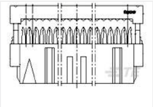
TE 产品编号4-215882-0 40 WAY BLACK MK II RECP
