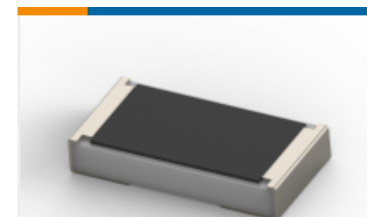
TE 产品编号2-2176231-6 SMD 功率电阻器：3 瓦特，1% Tol
