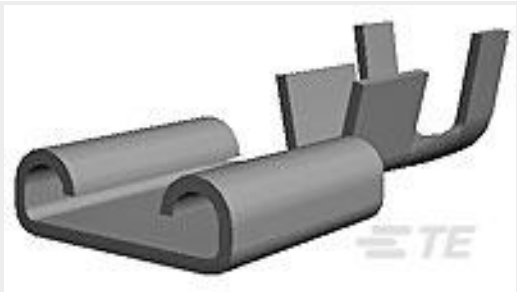
TE 产品编号280001-9 250 FASTON,REC.,14-17 AWG,TPBR
