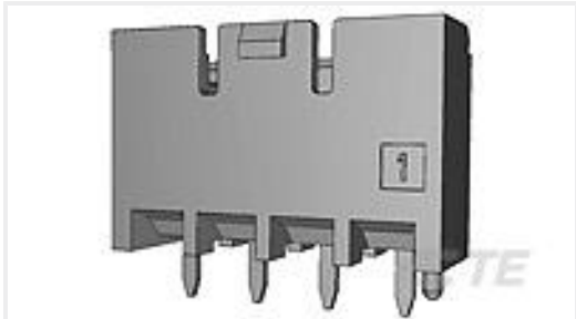
TE 产品编号2-1376421-3 10mm B-T-W Conn. 2P HDR ASSEMB
