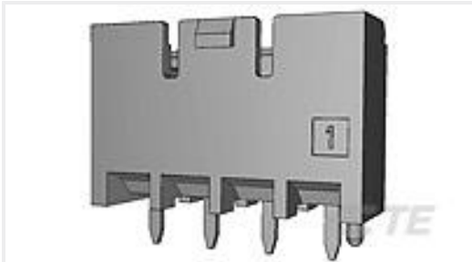
TE 产品编号1-1376384-2 5mm B-T-W Conn. 4P HDR ASSEMBL
