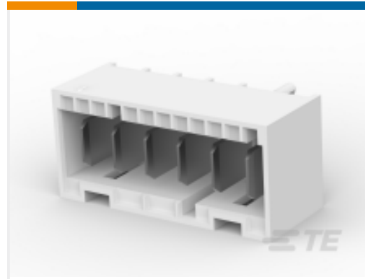
TE 产品编号 1-1971845-6 6P, RAST 5 Tab Header, THV
