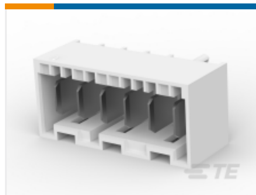
TE 产品编号 7-1971845-6 6P, RAST 5 Tab Header, THV
