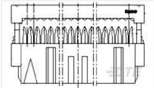
TE 产品编号1-215911-6 16 WAY BLACK MK II RECP
