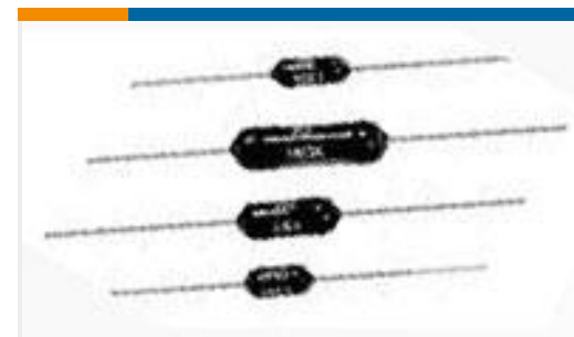
TE 产品编号7-1879693-3 H8 604R 0.1% 100PPM
