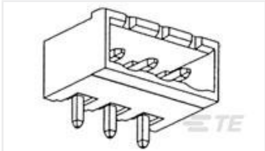
TE 产品编号 282818-2 TERMI-BLOK HEADER, ASSY90 2P.1
